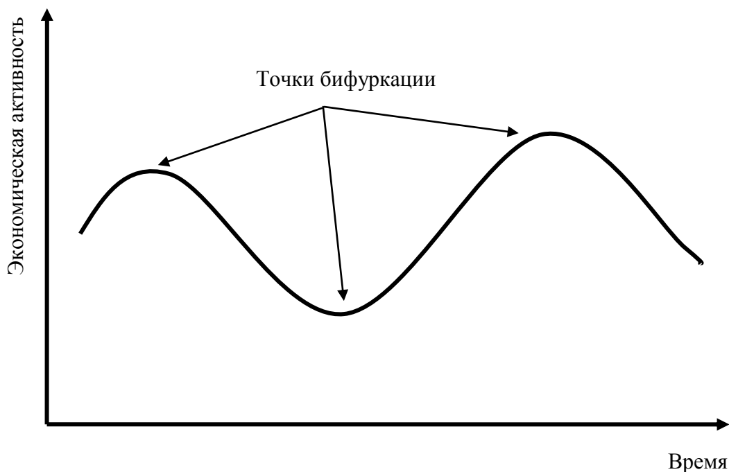
Рис. 3. Точки бифуркации
