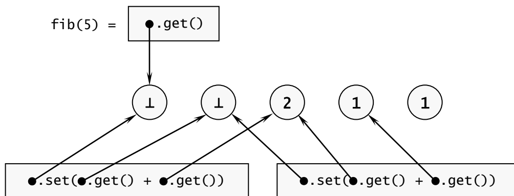
Рис. 4. Состояние вычисления fib(5) , после того как рекурсивная функция fibRec отработала, но оставила незавершившиеся сопрограммы, созданные операторами launch . Часть из них выполнялась и заполнила три монотонных объекта LongM значениями 2 = \text{fib}(2) , 1 = \text{fib}(1) , 1 = \text{fib}(0) . Две другие изображены прямоугольниками с выражениями u.set(v.get() + w.get()) со ссылками на объекты на местах переменных u , v , w . Объекты класса LongM изображены кругами, где знак 1 обозначает «неготовое» состояние, число – значение поля value .
